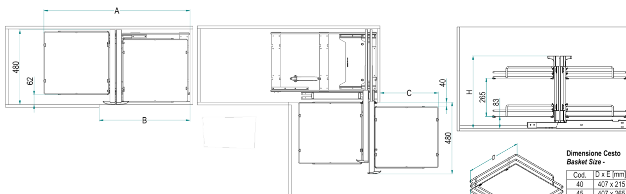
Compact 2 - Uniwersalny (L/P) mechanizm narożny pełen wysuw 839BE
