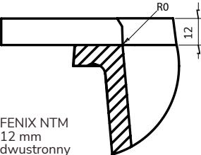
Szafka standardowa Montaż podblatowy do blatu 12mm
