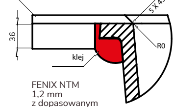
Szafka standardowa Montaż podblatowy do laminatu 1.2mm
