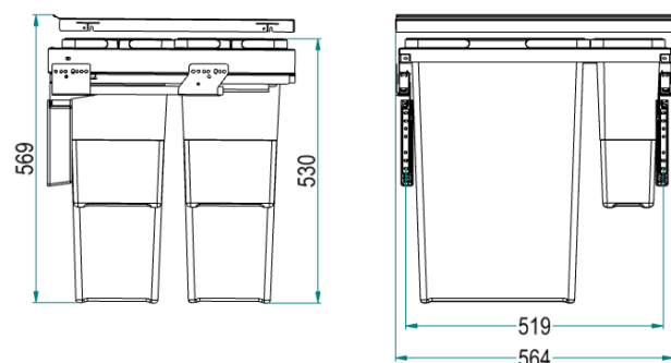
POJEMNIK NA ODPADKI DO SZAFEK O SZEROKOŚCI 60 CM
